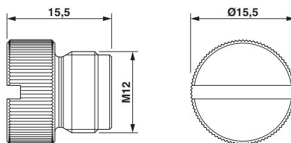
尺寸图
