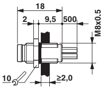
尺寸图
