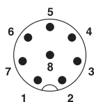
M12针式连接器引脚分配, 8芯, A编码, 插头侧视图
