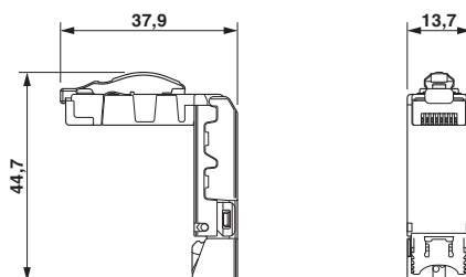
尺寸图
