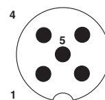
M12针式连接器引脚分配, 5芯, A编码, 插座侧视图
