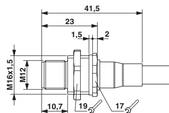
尺寸图
