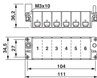
尺寸图
