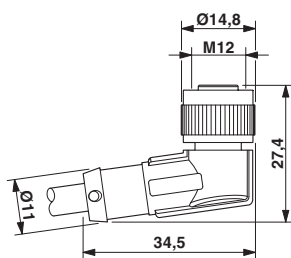
尺寸图
