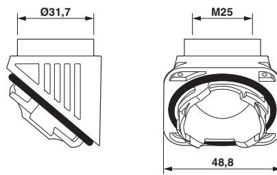
尺寸图
