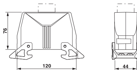
尺寸图
