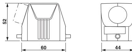
尺寸图
