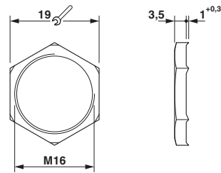
尺寸图
