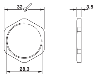
尺寸图
