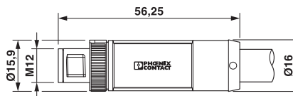
尺寸图
