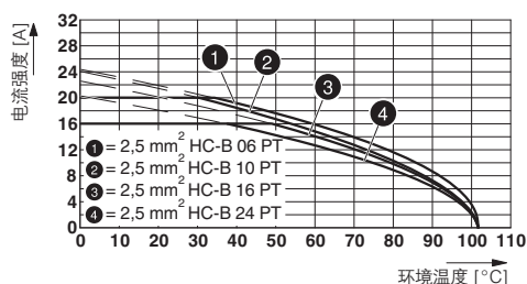
2.5 mm² 电缆的衰减曲线图
