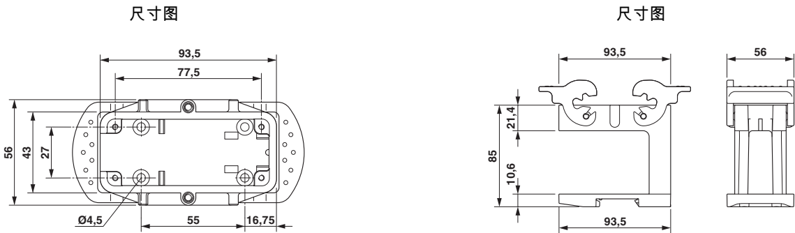
尺寸图
