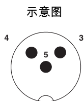
M12针式引脚分配, 3芯, 阀插头
