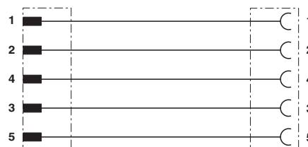
M12针式和M12孔式的触点分配
