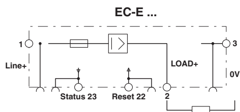
电路图
