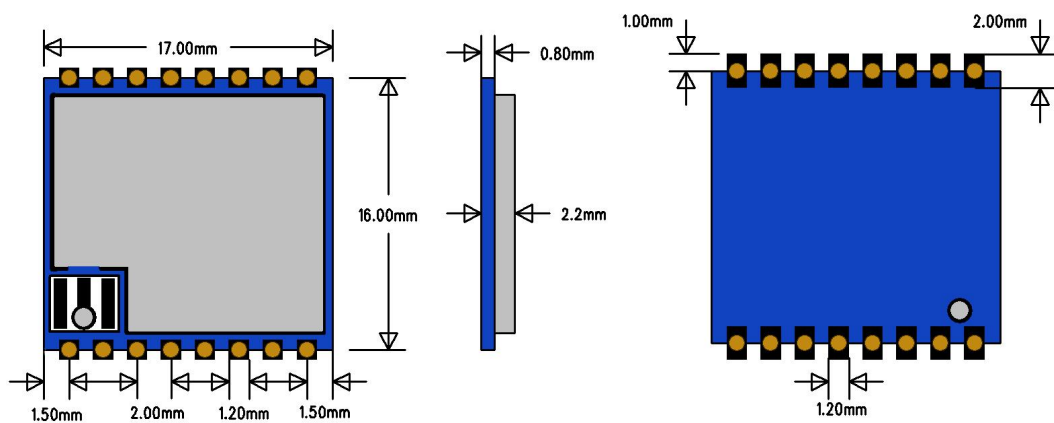
图 2. RC68A 尺寸图
