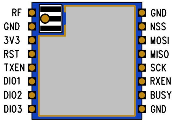
图 3. RC68A 引脚定义图 (Top View)
