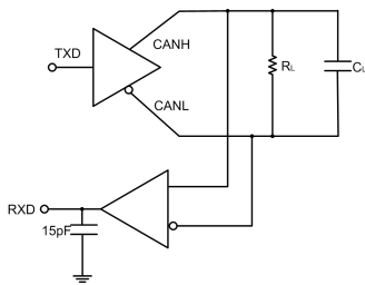
图13.传输特性测试电路
