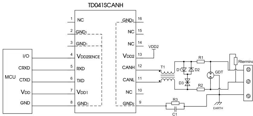
图 17. 端口保护推荐电路
