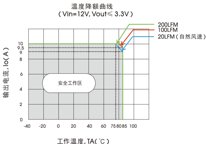
K12T-10A 系列温度降额曲线
