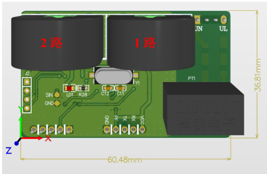
图 2.1 外形尺寸图 (单位: mm)
