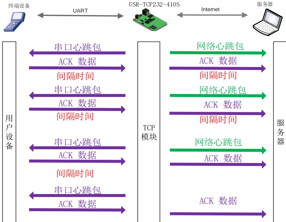
图 27 心跳包功能示意图
