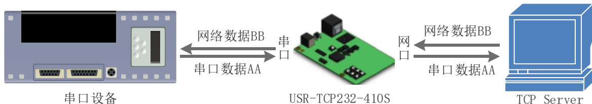
图 13 TCP Client 模式说明
