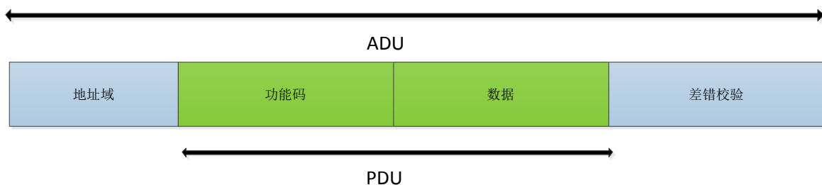
图 35 Modbus RTU 帧
