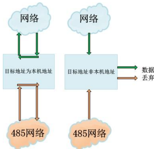
图 18 从机模式数据流向图
