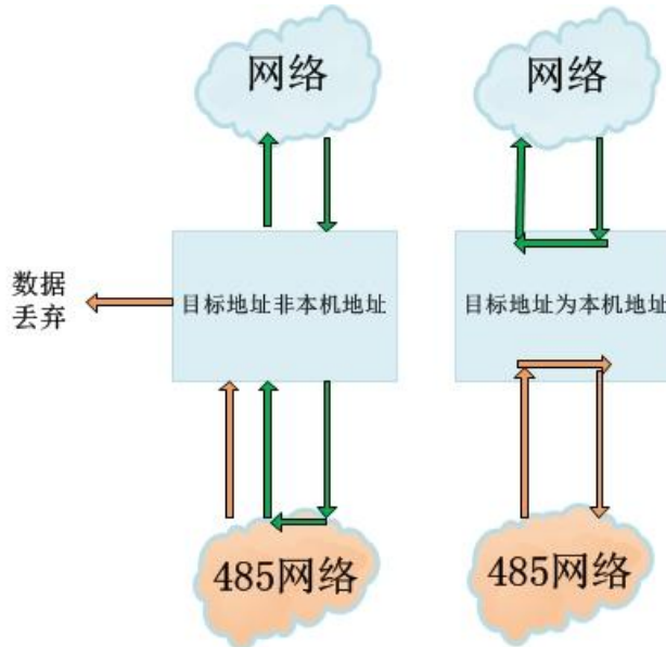
图 17 主机模式数据流向图
