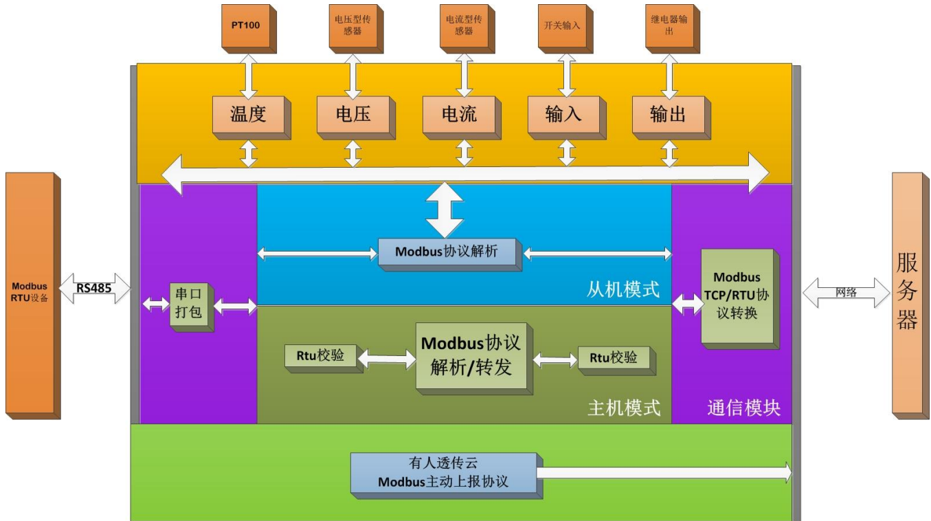
图 16 USR-IO424T-EWR 功能框图
