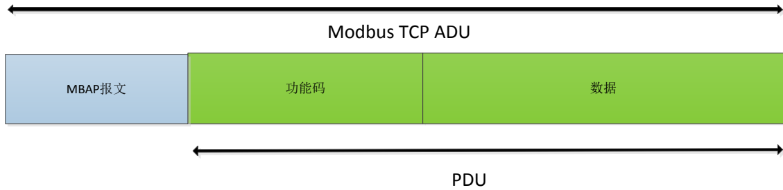
图 36 Modbus TCP 帧
