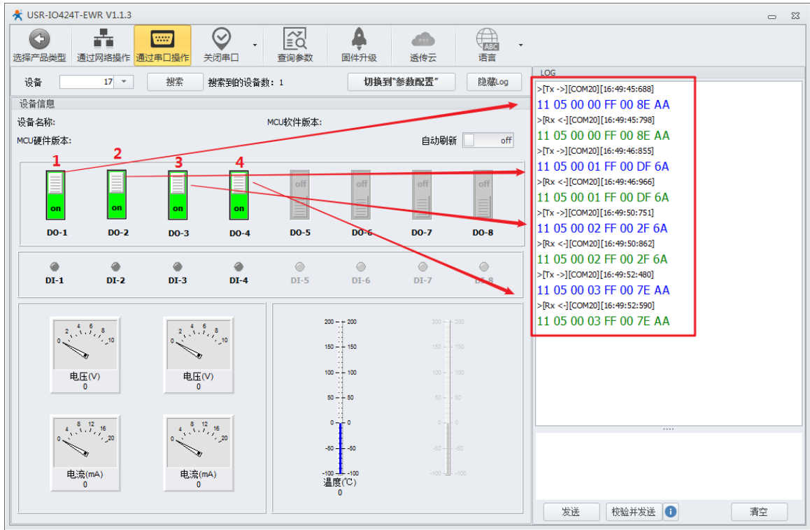
图 5 改变输出
