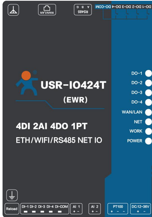
图 14 USR-IO424T-EWR 硬件接口示意图
