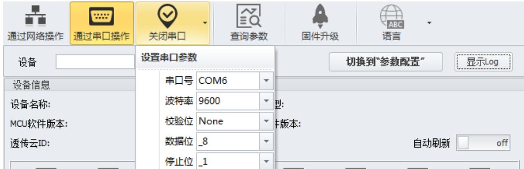
图 3 串口参数
