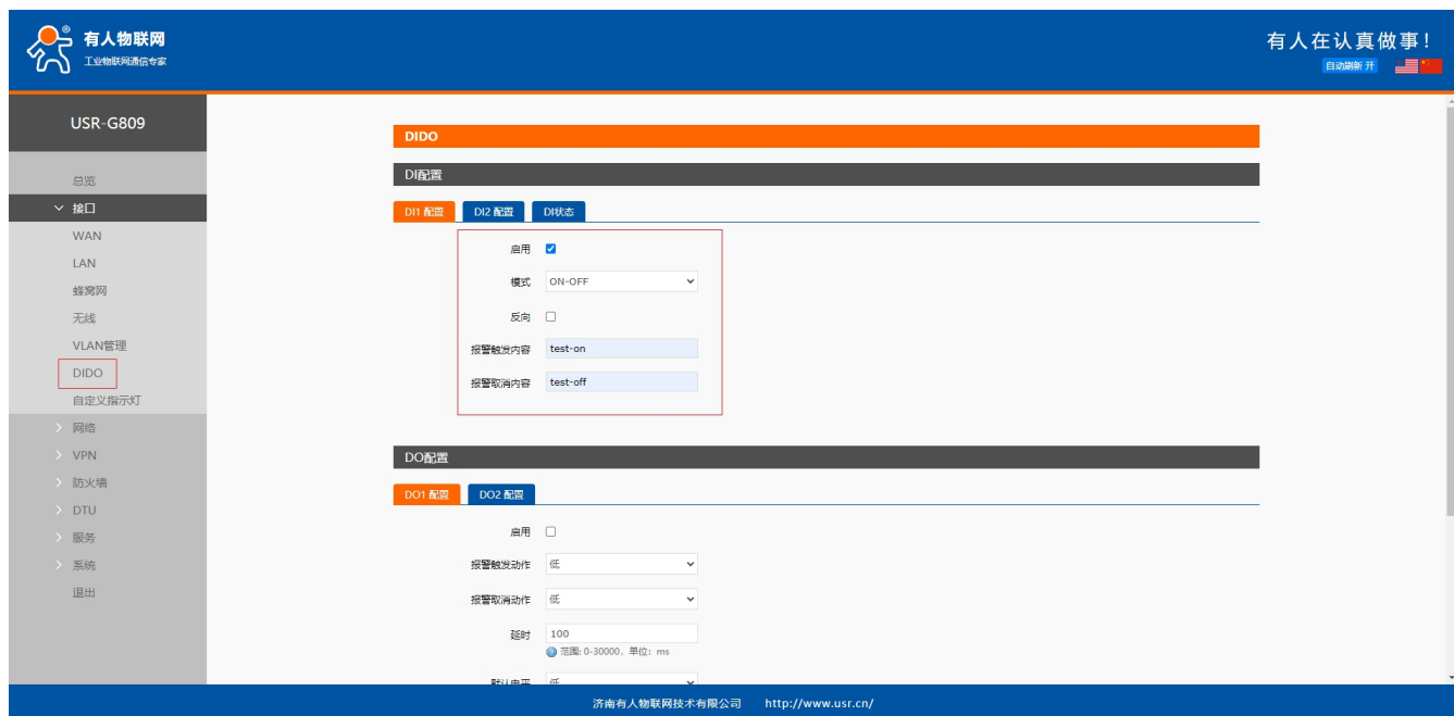
图 125 DI1 配置界面
