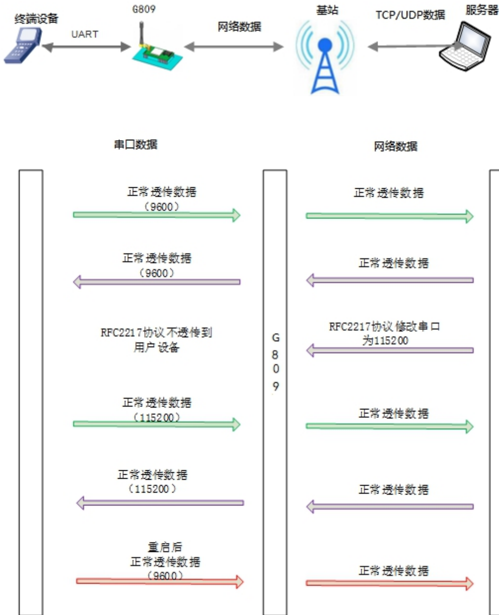
图 79 类 RFC2217 功能示意图
