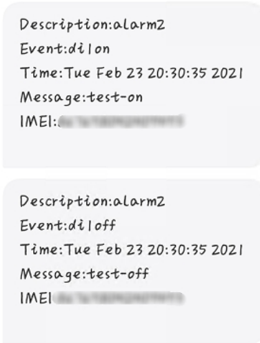
图 130 DI 动作时接收到的短信
