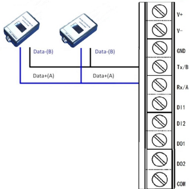
图 74 485 接线示意图
