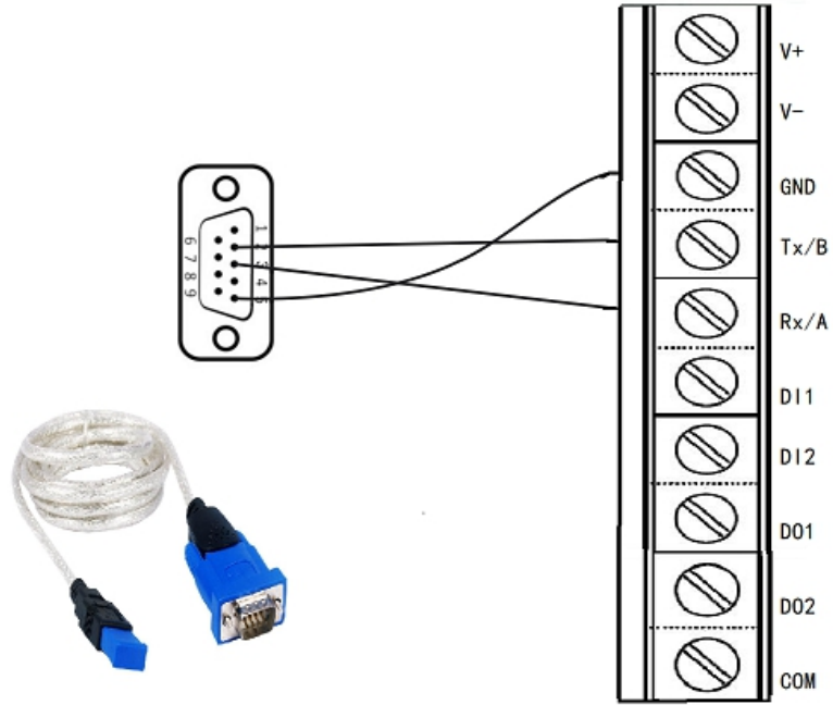
图 73 232 接线示意图
