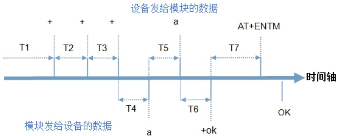
图 144 切换指令模式时序
