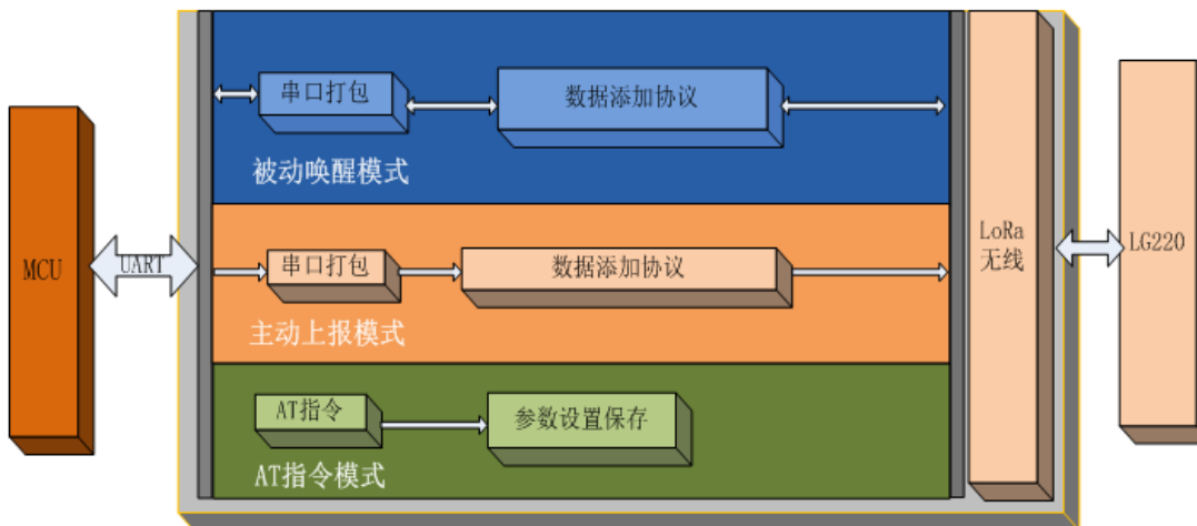
图 3 功能框图
