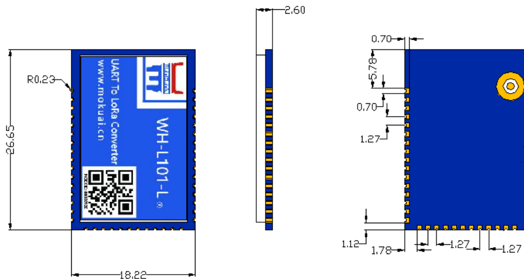
图 1 WH-L101-L 尺寸图
