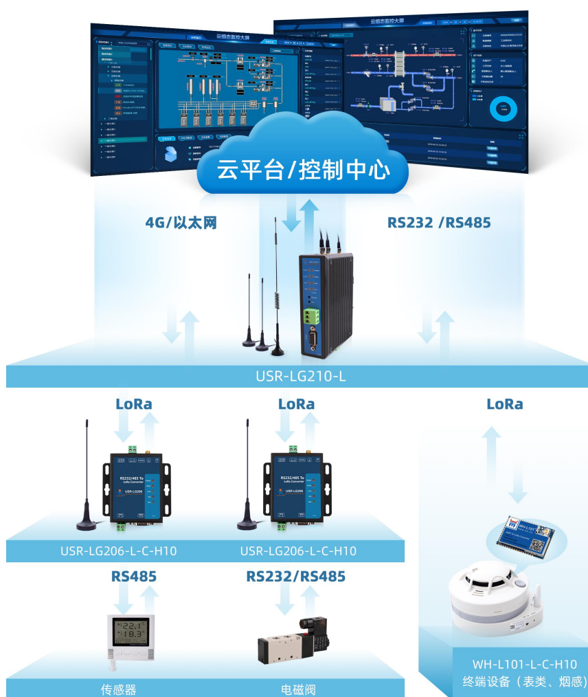
图 1.1 USR-LG210-L 应用框图
