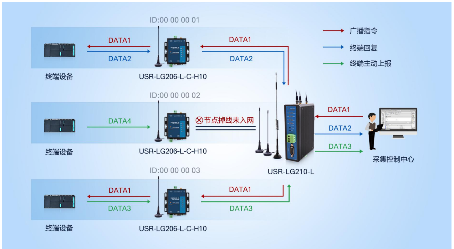
图 2.18 通信过程
