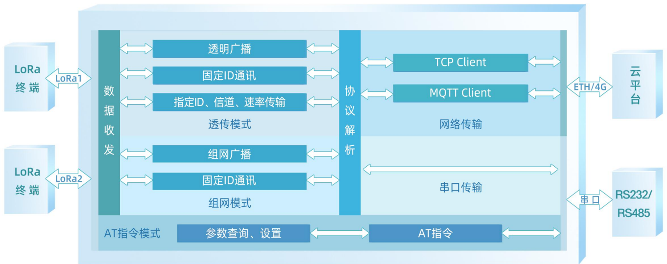
图 2.1 功能框架图
