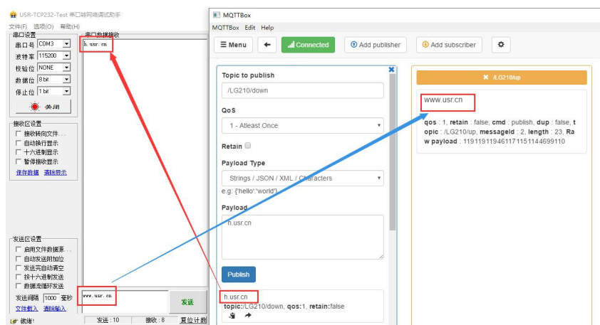
图 3.15 MQTT 通信过程
