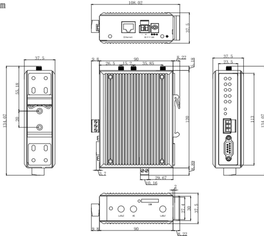
图 1.2 外观尺寸图
