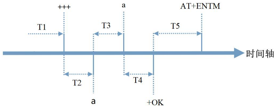
图 4.1 AT 指令模式切换时序
