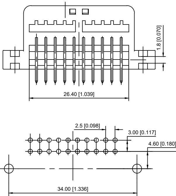
SEC:A - A
