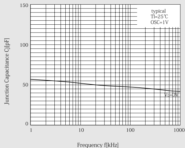
接合容量 Junction Capacitance
