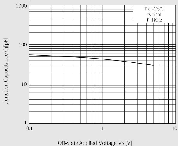
接合容量 Junction Capacitance
