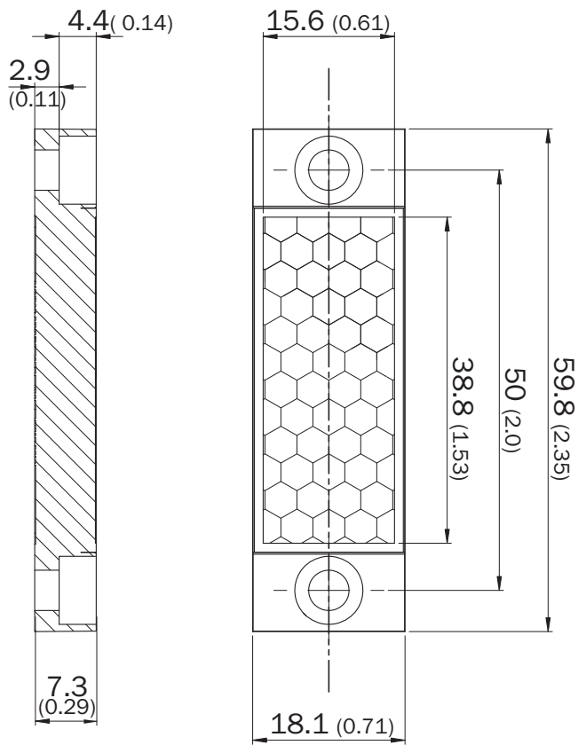
尺寸图 (尺寸单位: mm)
