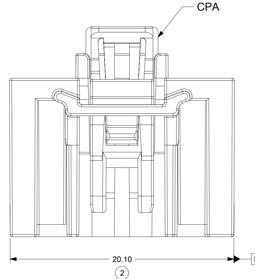
8CKT USCAR COMPATIBLE RECEPTACLE W/CPA
