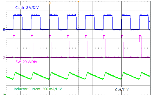
LMR38010-Q1 V_{OUT} = 5\text{ V} 400 kHz
