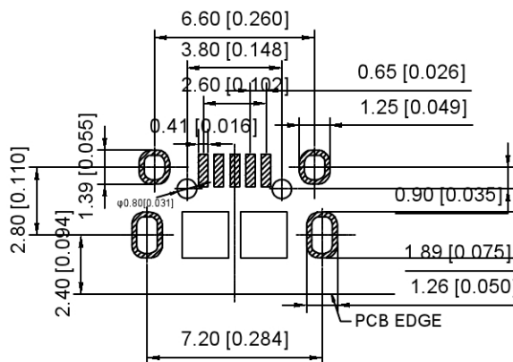
P.C.B.Land Pattern
