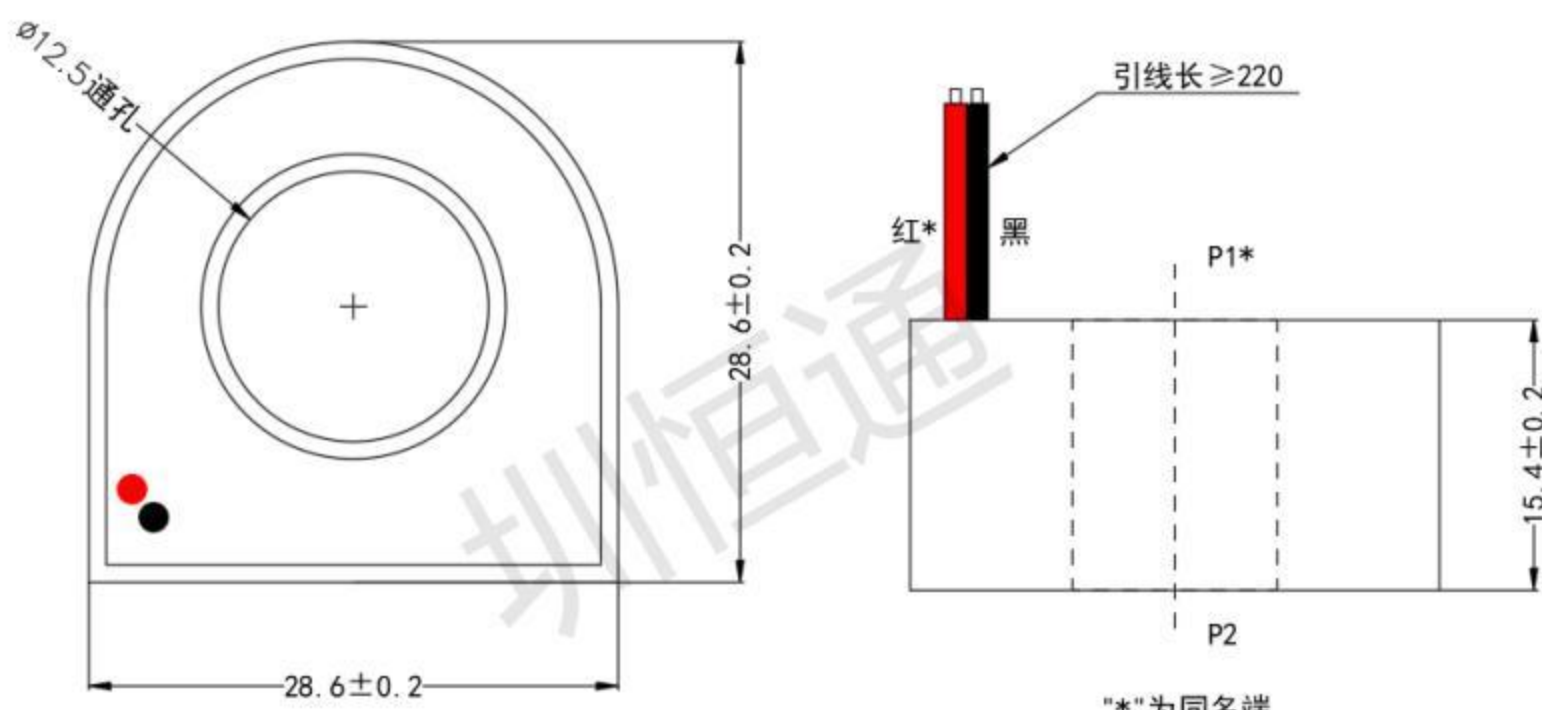
主视图
