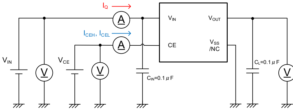
Test CIRCUITS①
