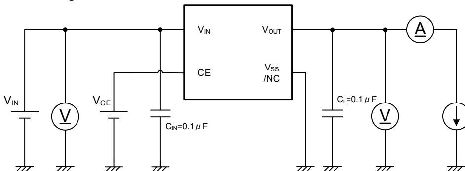
Test CIRCUITS④
