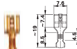
FSH6,3x0,8
