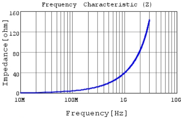
LQP03TN6N2H02 |Z|
