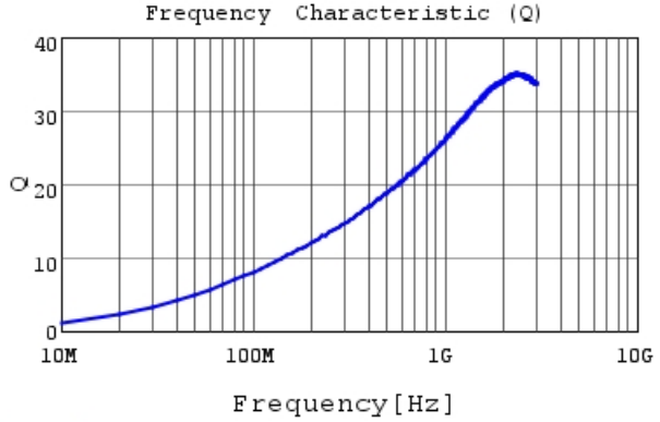
LQP03TN6N2H02 Q
