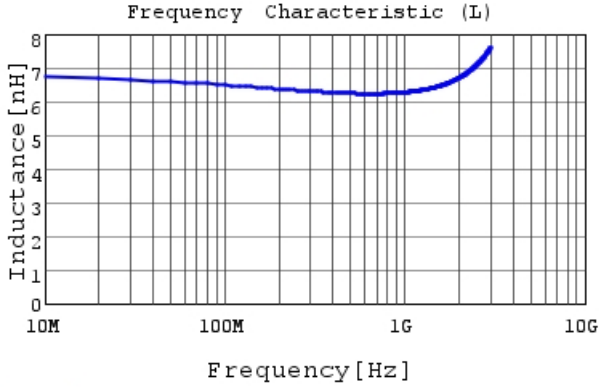
LQP03TN6N2H02 L
