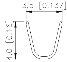
SECTION:A-A SCALE: 1:1
