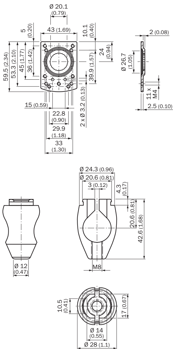
尺寸图 (尺寸单位: mm)
