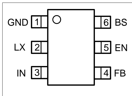
SOT23-6
