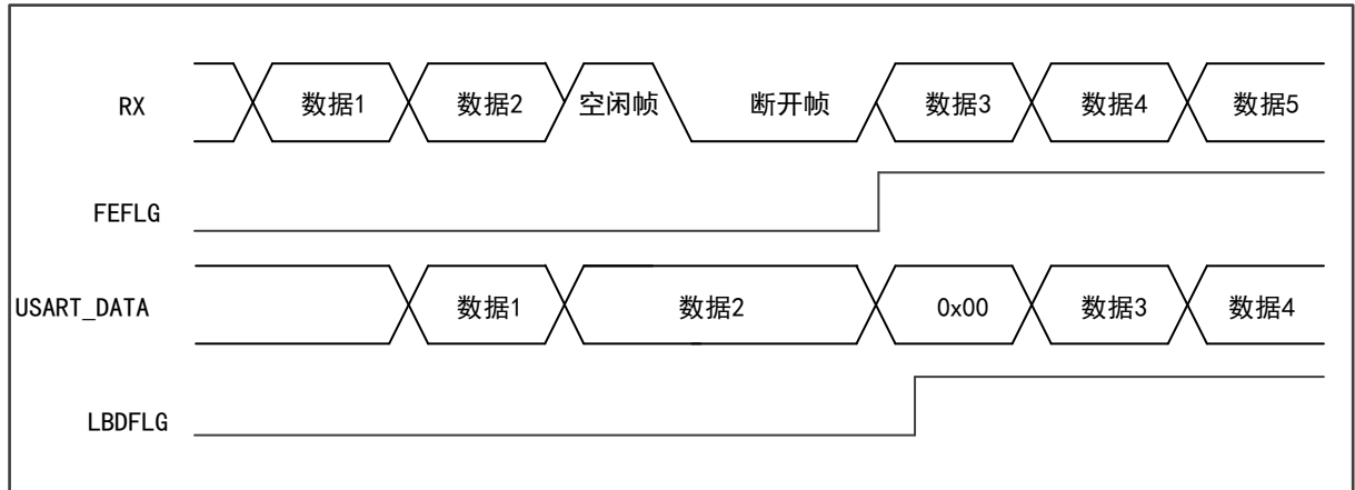
图 76 空闲状态检测断开帧
