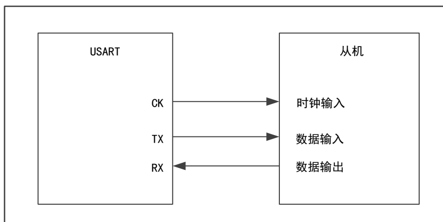
图 73 USART 同步发送的例子
