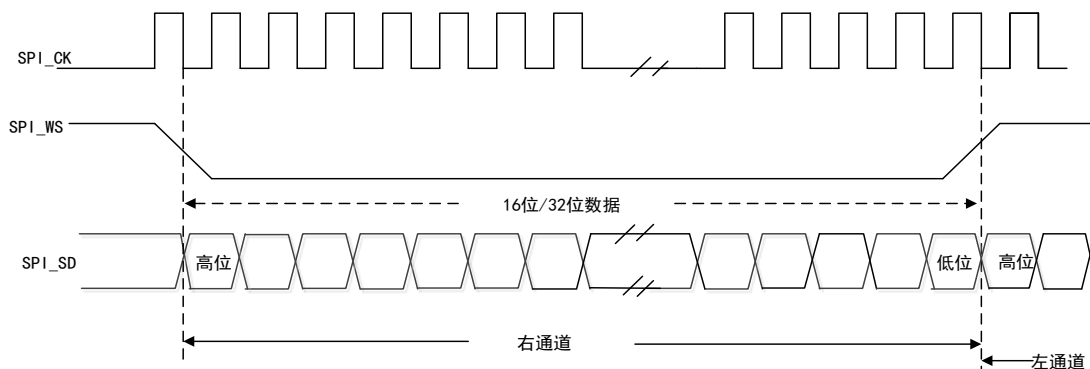
图 100 LSB 对齐标准波形（16/32 位数据）
