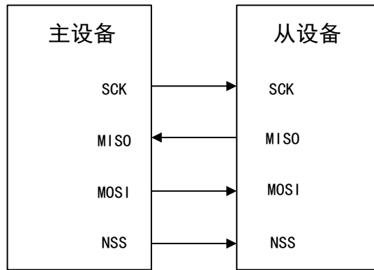
图 91 半双工模式连接（主机用来接收，从机用来发送）
