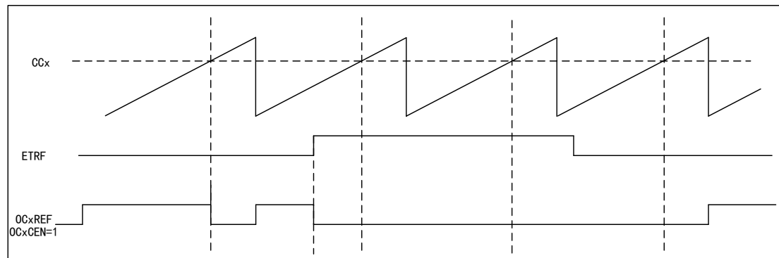
图 37 OCxREF 时序图
