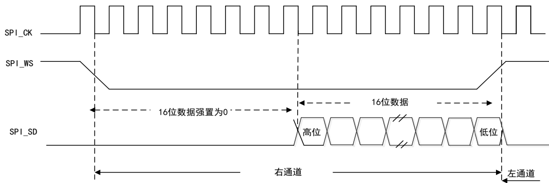
图 102 LSB 对齐标准下（16 位扩展至 32 位）
