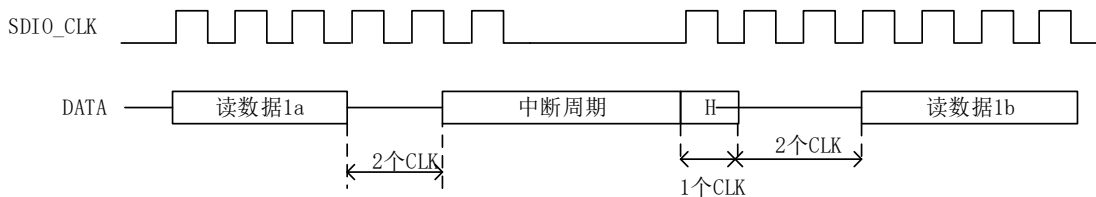
图 121 通过停止 SDIO_CLK 的读等待操作
