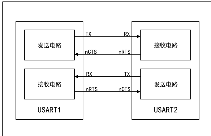
图 80 两个 USART 之间的硬件流控制
