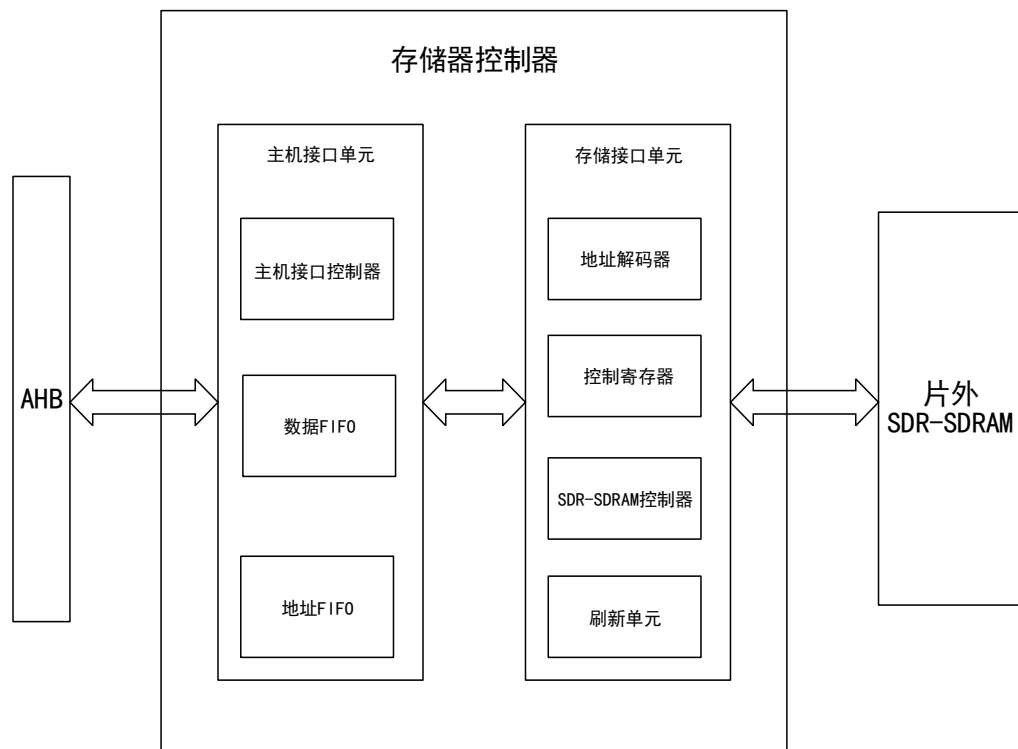
图 3 DMC 结构框图
