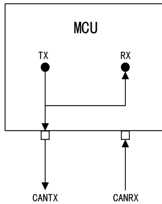
图 108 CAN 工作在环回模式
