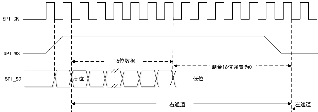
图 96 I2S 飞利浦协议波形（16 位扩展至 32 位）
