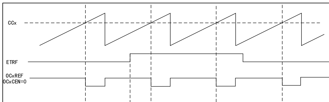
图 52 OCxREF 时序图
