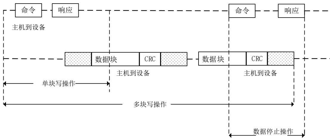
图 117 SDIO (多) 数据块写操作
