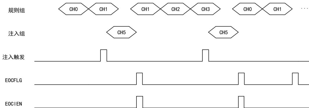
图 126 触发注入时序图
