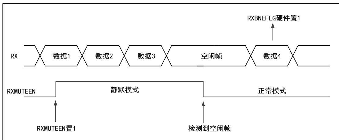
图 71 空闲总线退出静默模式
