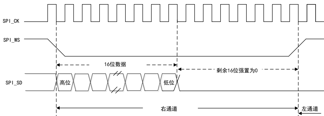
图 99 MSB 对齐标准波形（16 位扩展至 32 位）
