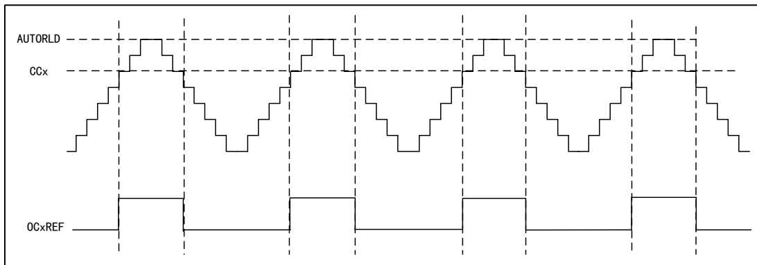
图 61 PWM2 中央对齐模式的时序图
