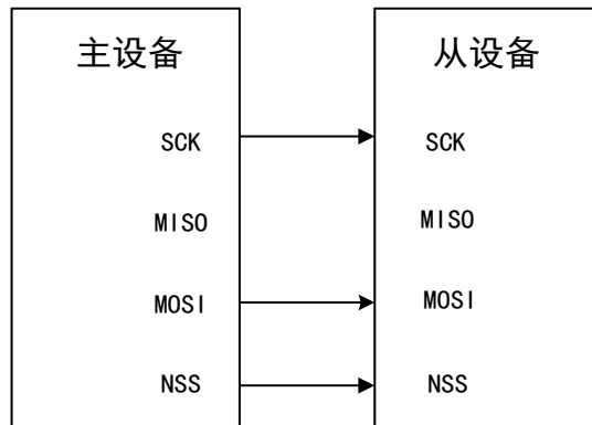
图 92 半双工模式连接（主机只发送，从机接收）
