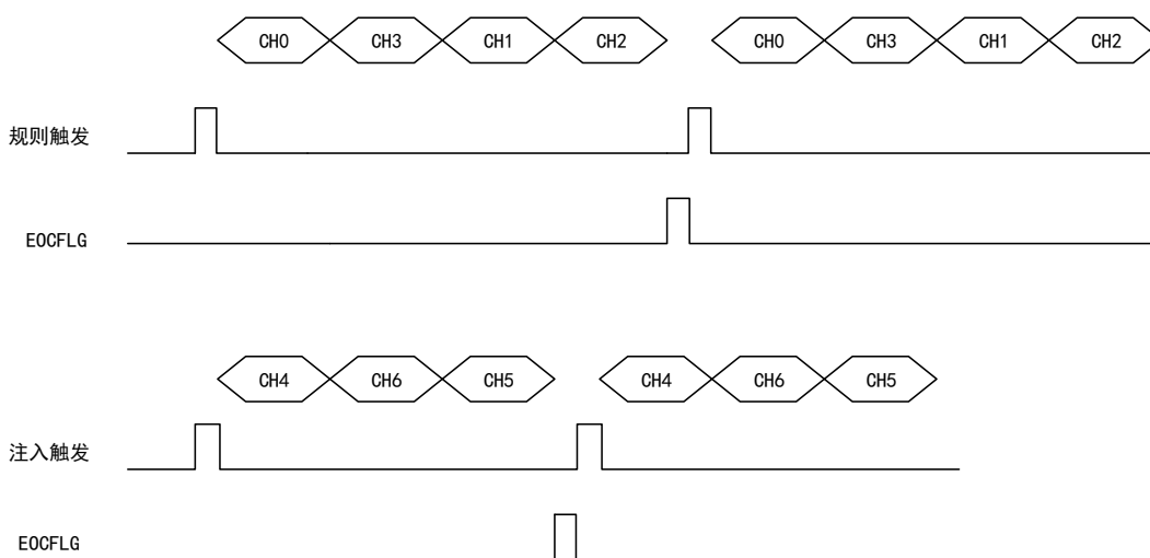
图 124 扫描模式时序图
