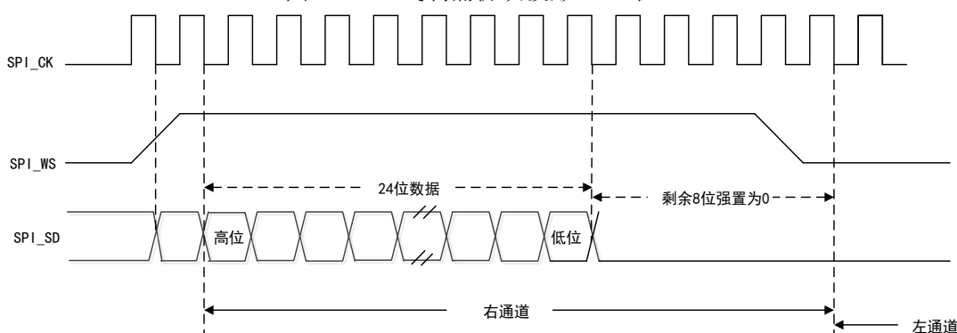
图 95 I2S 飞利浦协议波形（24 位）
