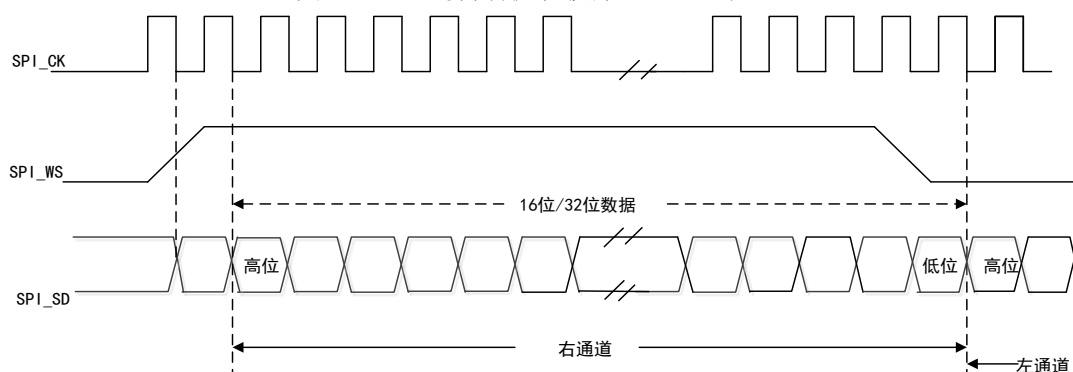
图 94 I2S 飞利浦协议波形（16/32 位）
