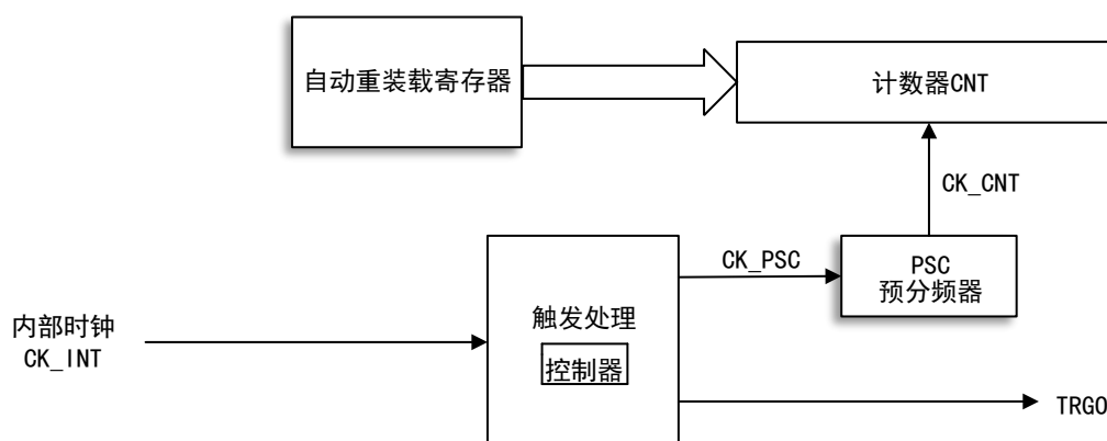
图 63 基本定时器结构框图
