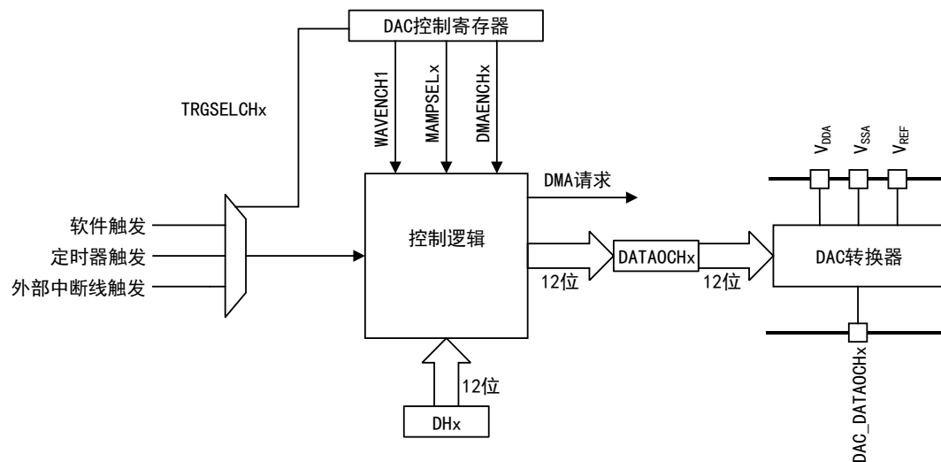
图 128 DAC 结构框图
