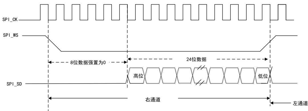
图 101 LSB 对齐标准波形（24 位数据）
