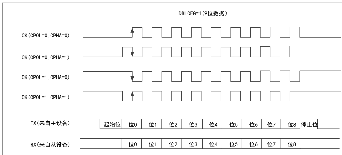
图 75 USART 同步发送时序图 (DBLCFG=1)
