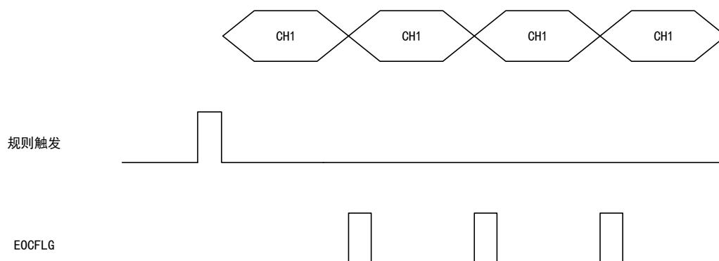
图 123 连续转换模式时序图
