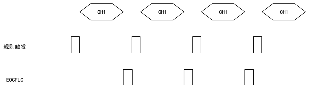
图 122 单次转换模式时序图
