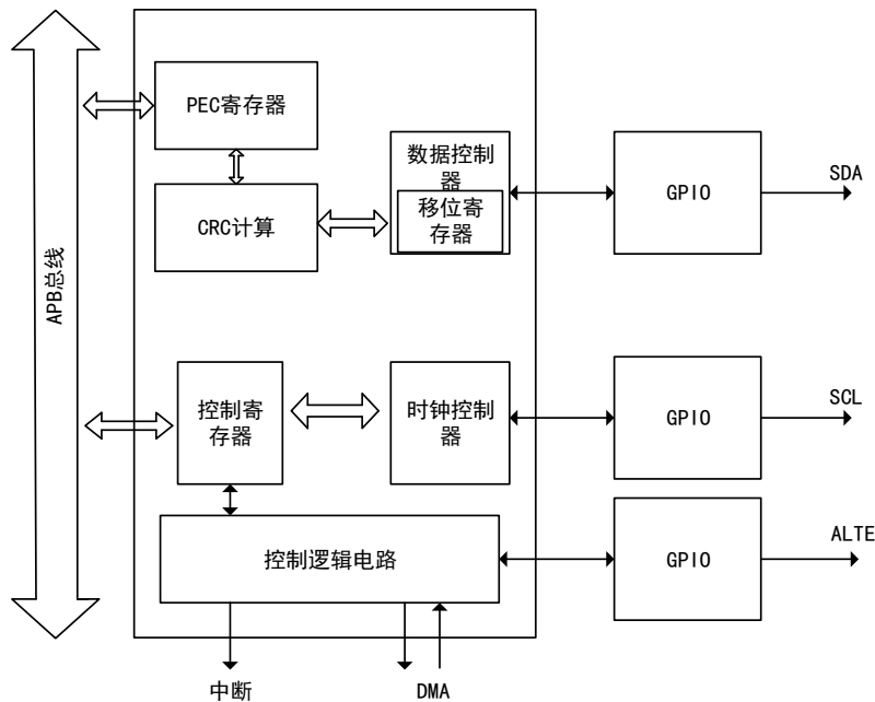
图 82 I2C 功能结构图
