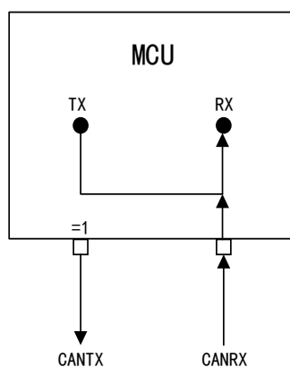
图 107 CAN 工作在静默模式
