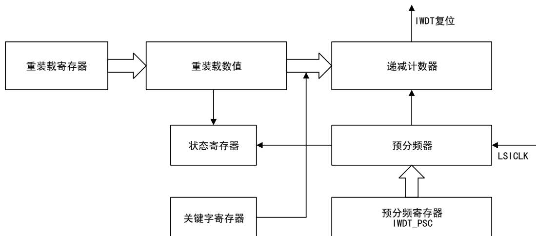
图 65 独立看门狗结构框图
