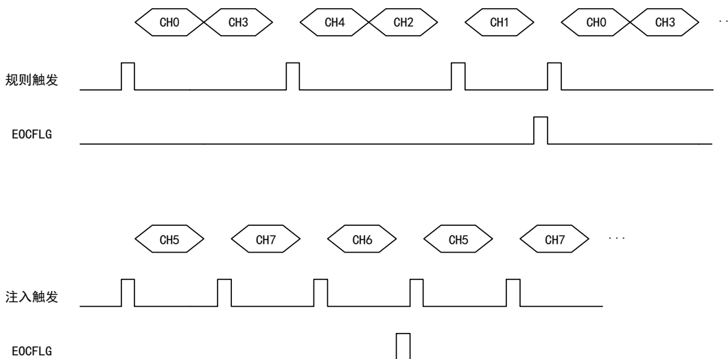
图 125 间断模式时序图
