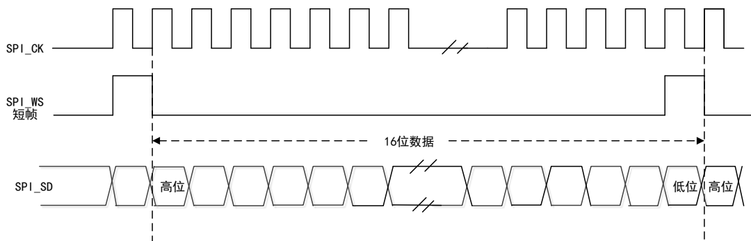
图 104 PCM 标准波形
