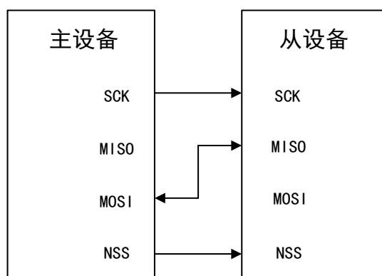
图 93 双向线连接
