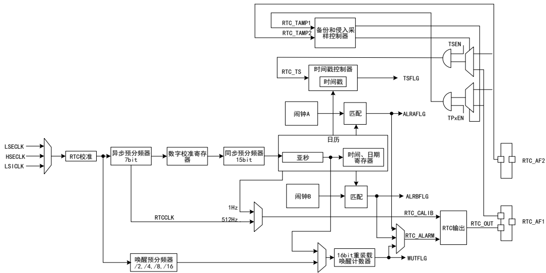
图 68 RTC 结构框图
