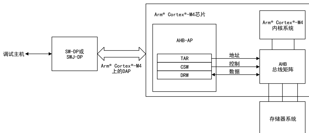
图 12 APM32F4xx 级别和 Arm® Cortex®-M4 级别的调试框图
