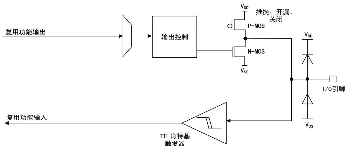
图 16 复用模式 I/O 结构
