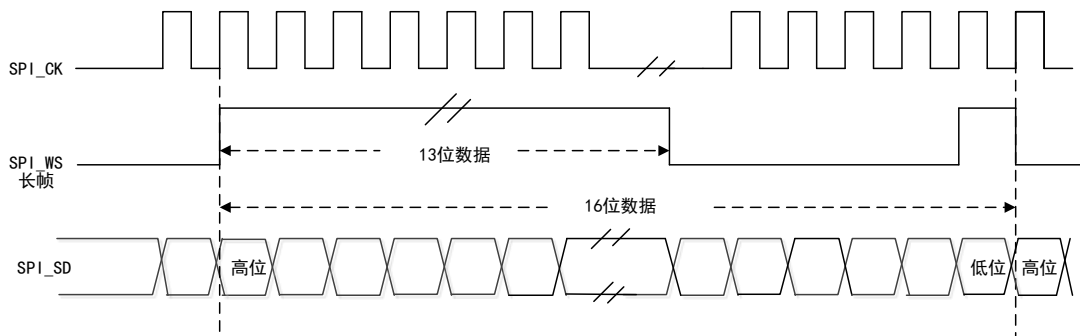
图 103 PCM 标准波形
