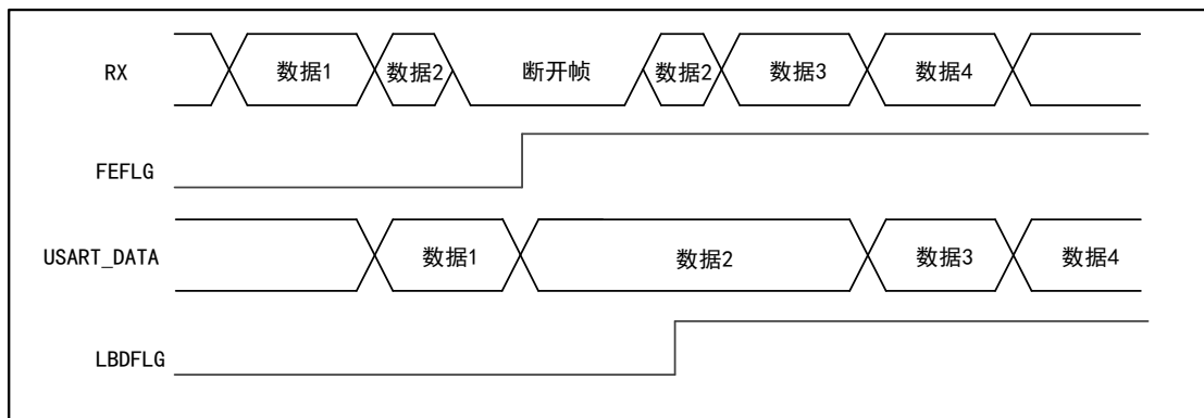
图 77 数据发送状态检测断开帧
