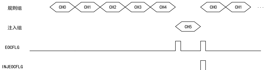
图 127 自动注入时序图
