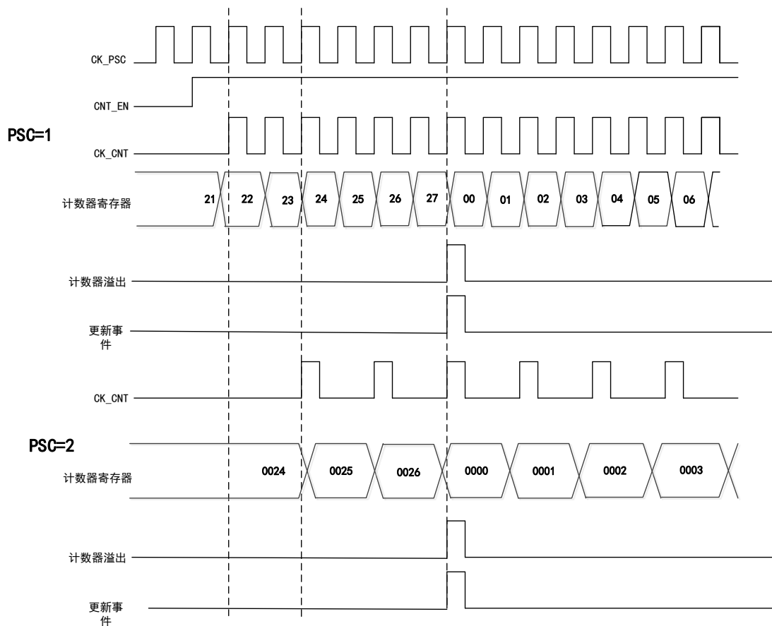
图 64 计数器时序图，内部时钟分频系数为 1 或 2
