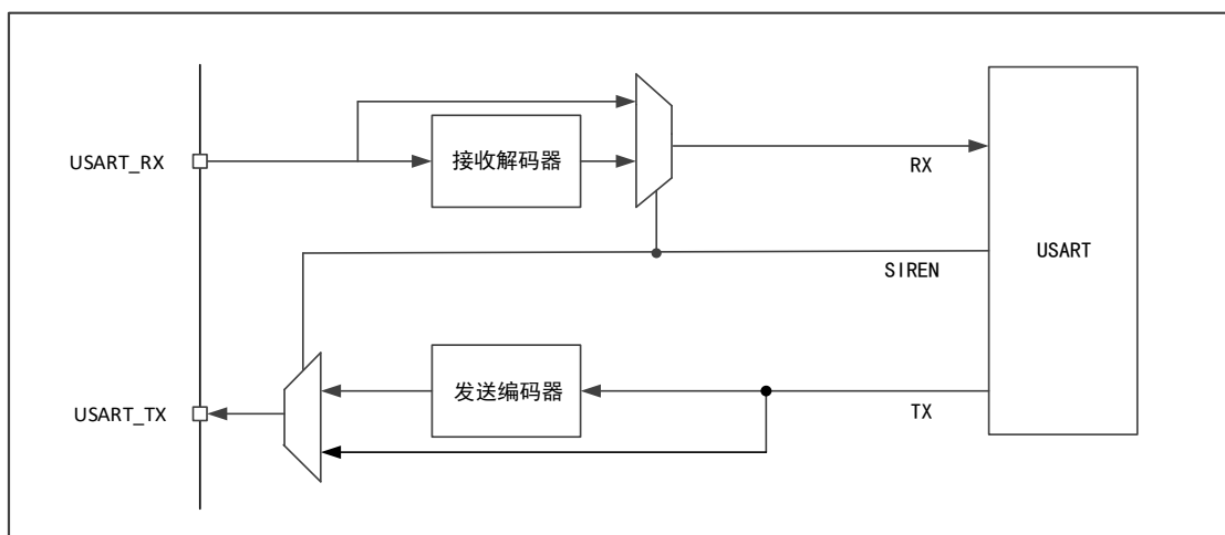
图 79 IrDA 模式框图
