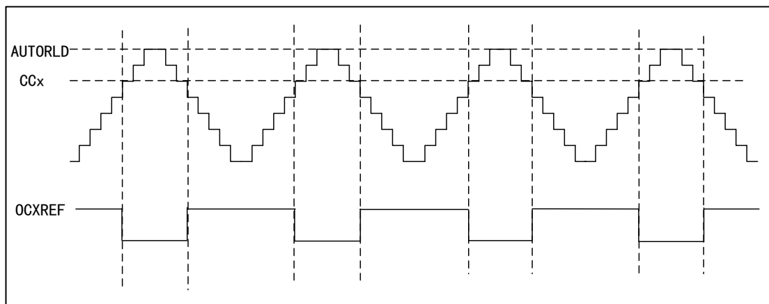
图 60 PWM1 中央对齐模式的时序图
