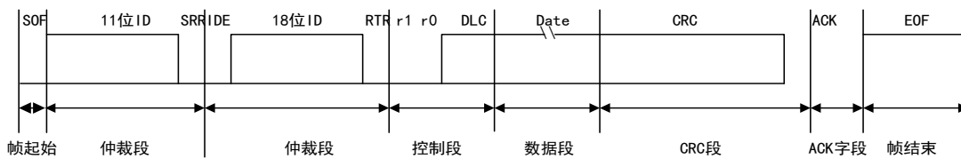
图 106 扩展数据帧
