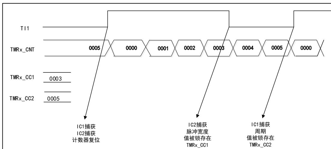
图 59 PWM 输入模式时序图
