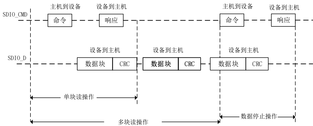
图 116 SDIO (多) 数据块读操作
