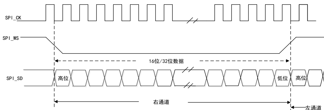
图 97 MSB 对齐标准波形（16/32 位数据）
