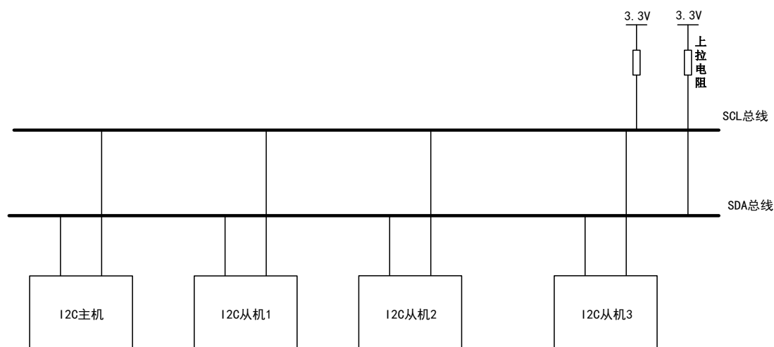
图 83 常见 I2C 通信连接图
