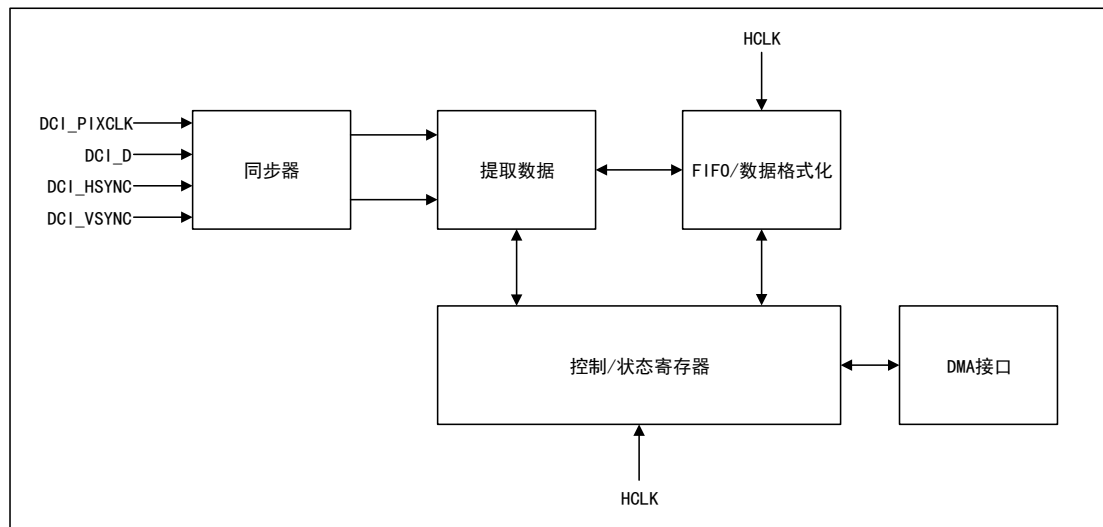
图 69DCI 结构框图
