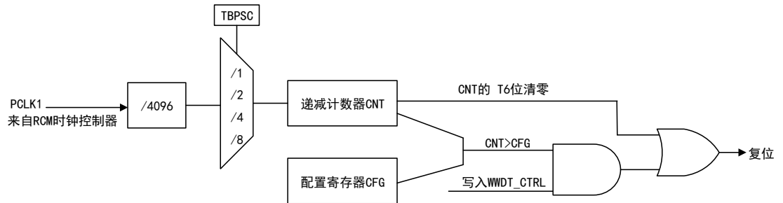
图 66 窗口看门狗结构框图
