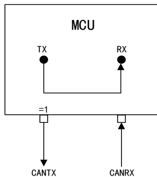
图 109 CAN 工作在静默环回模式
