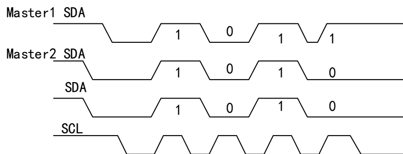
图 89 SDA 时序图
