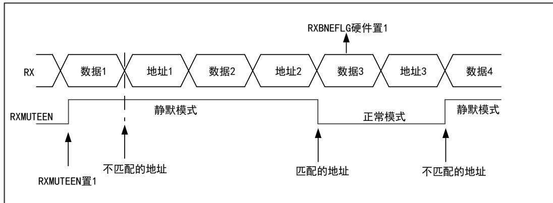
图 72 地址标记退出静默模式
