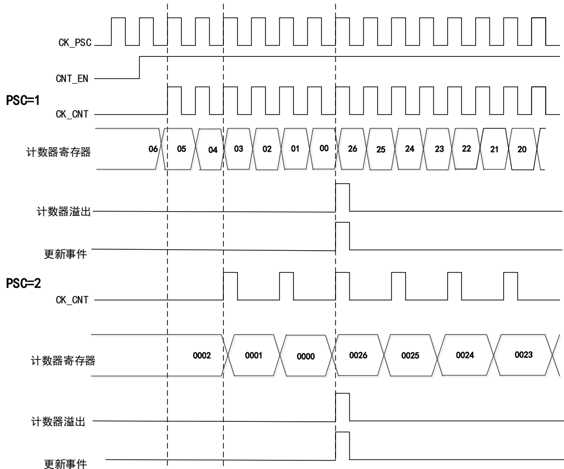
图 57 向下计数模式下，分频因子为 1 或 2 的时序图
