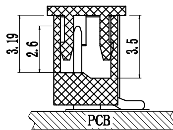
剖面 A-A
