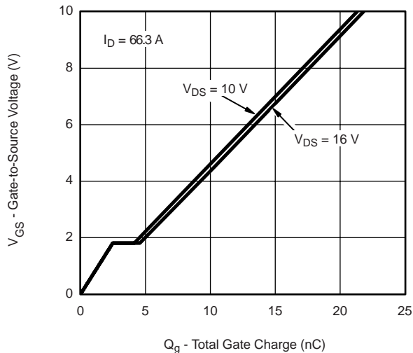
I_D = 66.3\text{ A} V_{DS} = 10\text{ V} V_{DS} = 16\text{ V} Gate Charge
