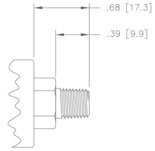
-4 1/8-27 NPT
