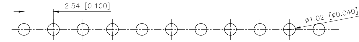
P.C.B LAYOUT
