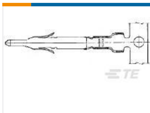
TE Part #170363-3 MINI UNIVERSAL M-N-L PIN LP
