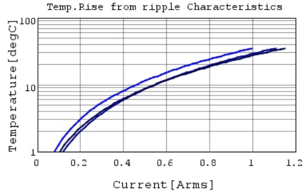
GRT033C71C104KE01 Temp.rise — 400kHz
