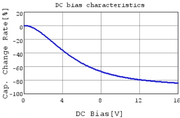
GRT033C71C104KE01 C-DC bias capchange, 25.0c
