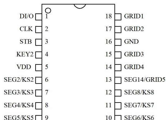
AIP1630 DIP-18
