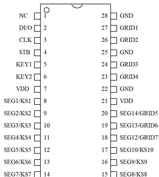
AIP1667 SOP-28
