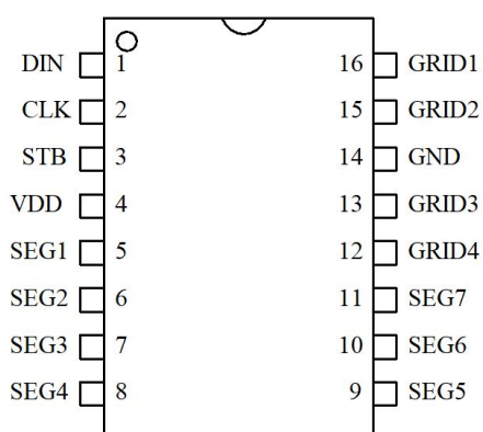
AIP1616 SOP-16
