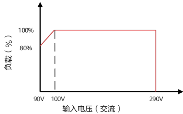
输入电压与输出功率降额
