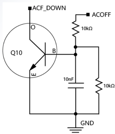
图 5-4 内部电路
