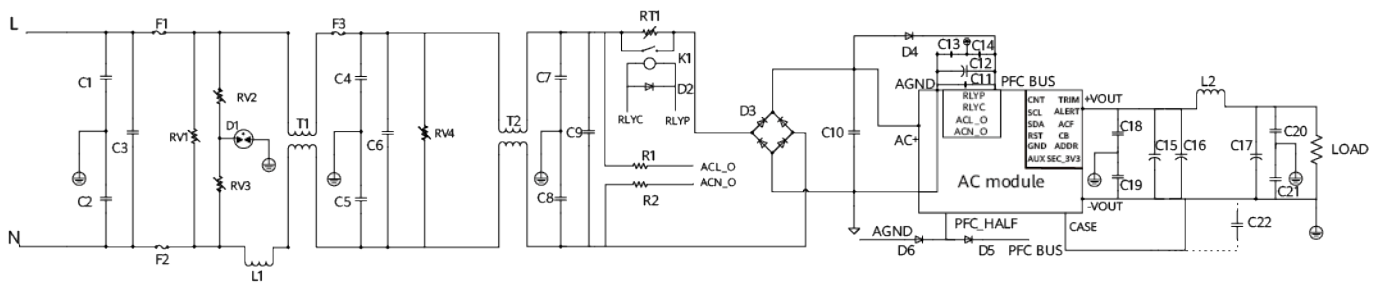
图 4-1 推荐电路
