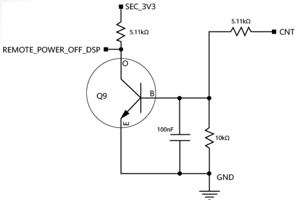
图 5-3 内部电路
