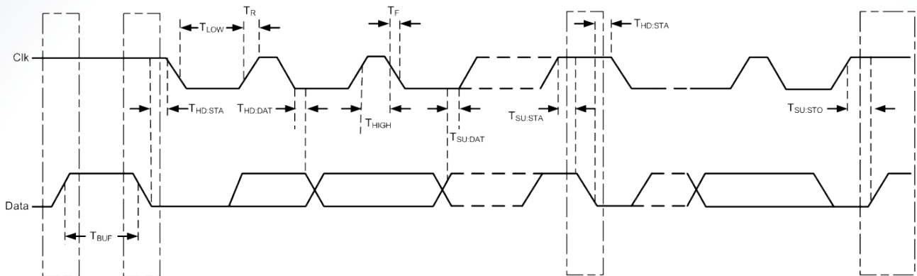
图 8-2 PMBus 时序
