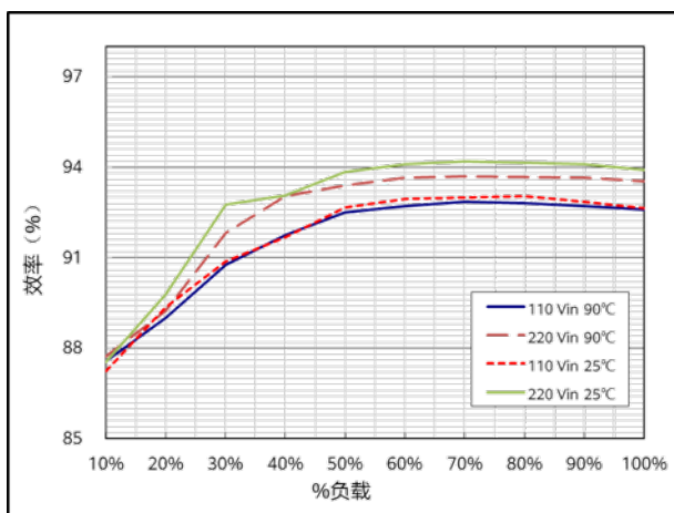
效率 ( V_{out}=42V , T=25^{\circ}C/90^{\circ}C )
