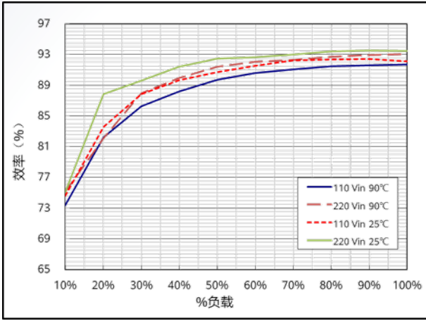
效率 ( V_{out}=55V , T=25^{\circ}C/90^{\circ}C )
