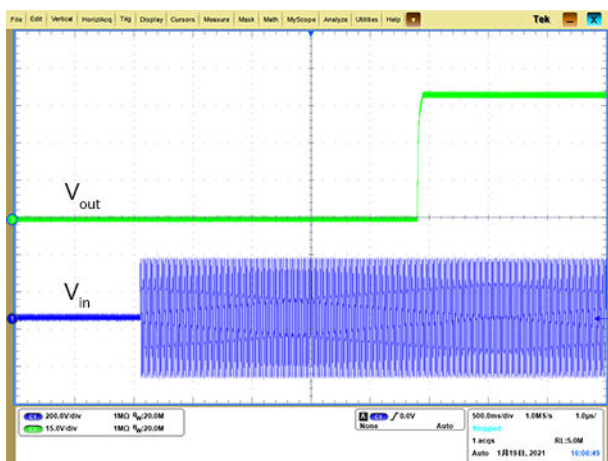
开机 ( V_{in}=220V AC, V_{out}=50V DC)
