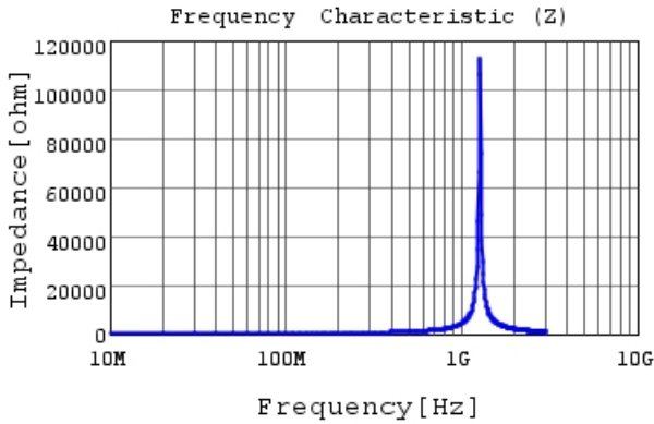
LQW18ASR27G00 |Z|
