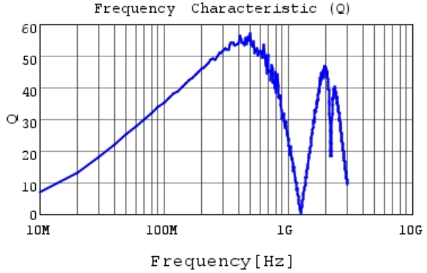
LQW18ASR27G00 Q
