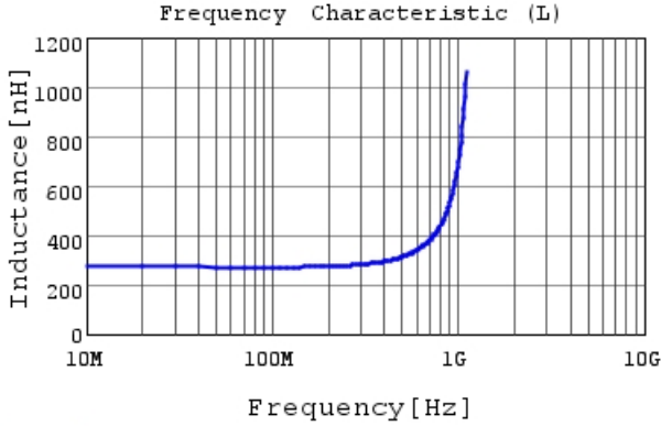
LQW18ASR27G00 L
